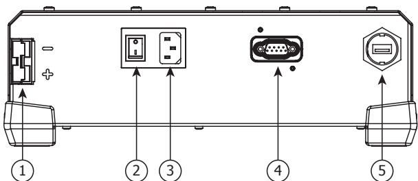
GYSFLASH 101.12 CNT
