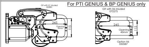
G9_X1 - 022881 8 bar / 550 daN
