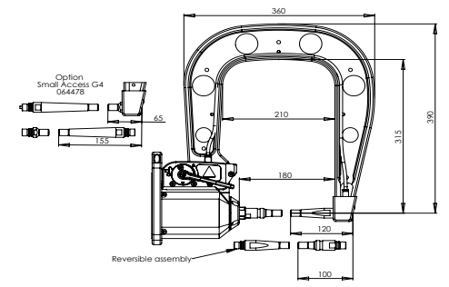
G14 - 080942 8 bar / 550 daN
