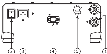
GYSFLASH 53.48 CNT
